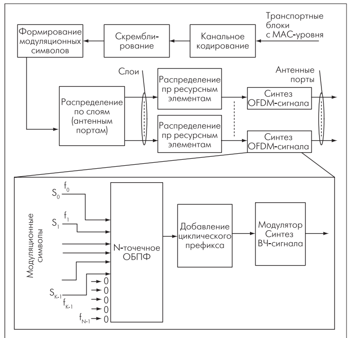
Рис.10. Схема формирования сигнала в нисходящем канале
