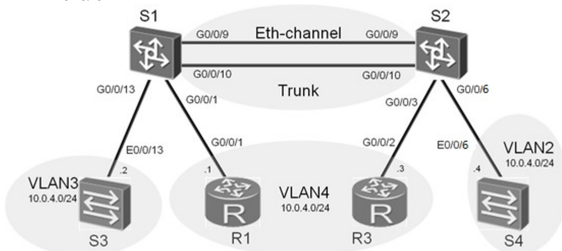
Рис 1.2 Топология VLAN
